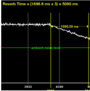
2. Mesure de durée de réverbération.
