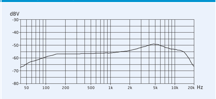
Courbe de réponse en fréquence MMD 845-1
