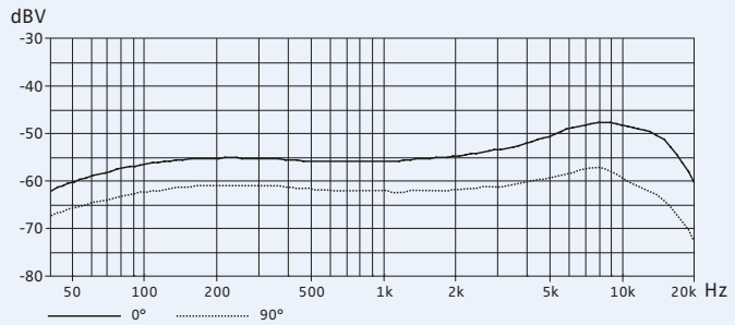
Courbe de réponse en fréquence MME 865-1
