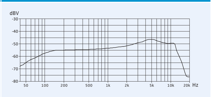
Courbe de réponse en fréquence MMD 835-1
