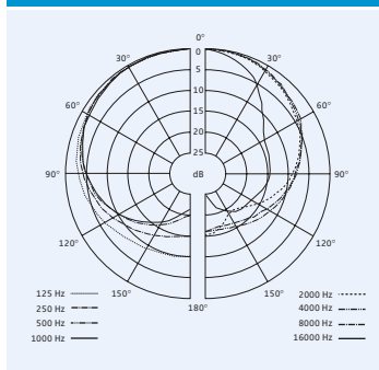
Diagramme polaire MMD 835-1
