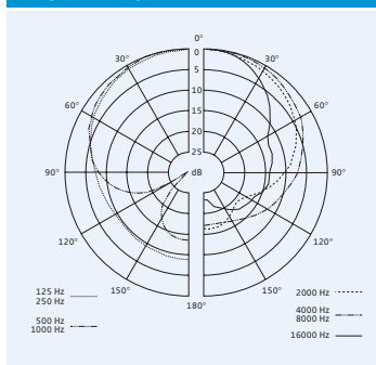
Diagramme polaire MMD 845-1
